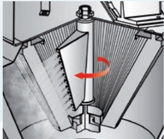
Rotating filter cleaning. Pulizia filtro rotante.
