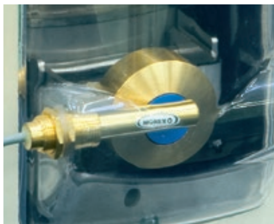
Discharging valve gravity sensor. Sensore valvola scarico a gravità.
